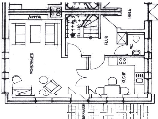
Grundriss EG
