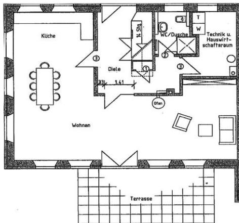
Grundriss EG
