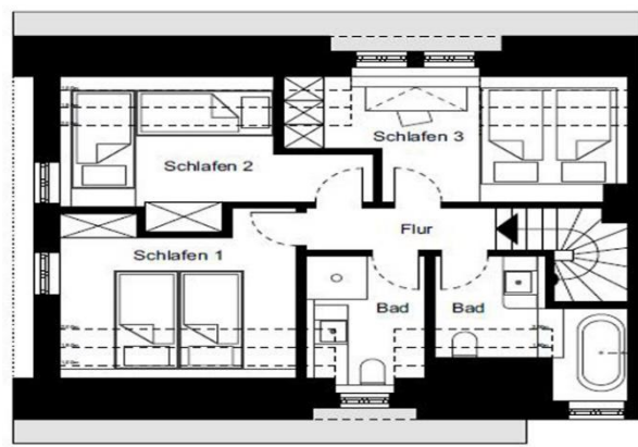
Grundriss Obergeschoss
