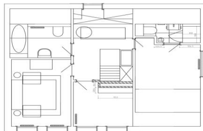
Grundriss OG
